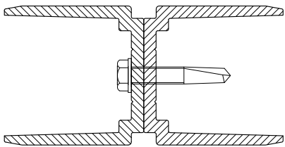
1-1 (разрез вкладыша)
